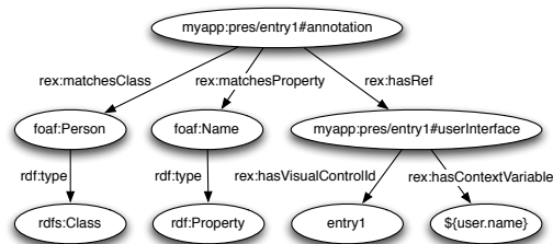
Figura 2: Grafo RDF que representa la metainformación de un control del formulario.
